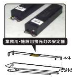
安定器
