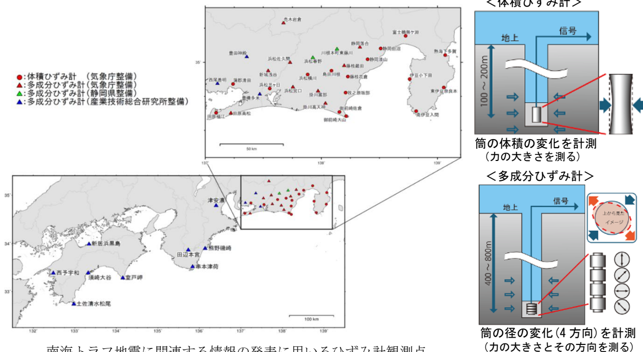
南海トラフ地震に関連する情報の発表に用いるひずみ計観測点
