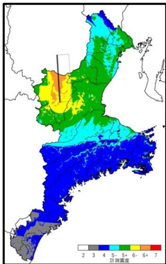
頓宮断層
