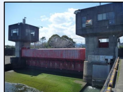
神内川防潮水門
