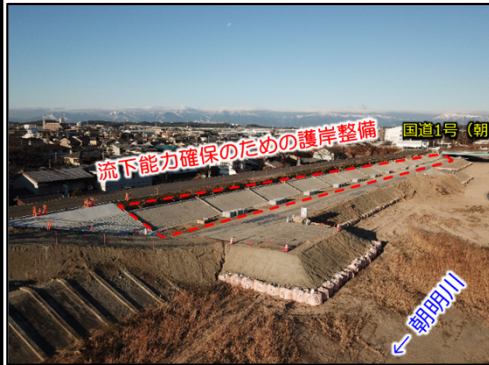
朝明川における護岸整備 （三重県）
