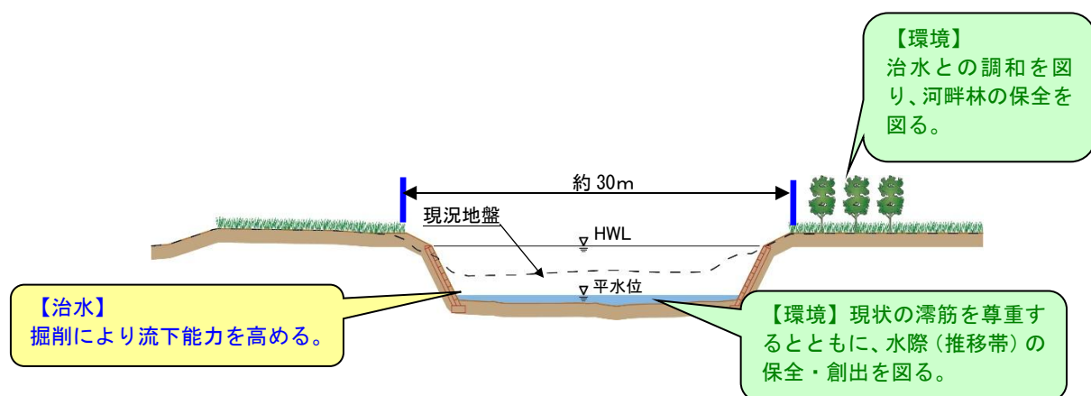
14km 付近の計画横断イメージ図 （横断形状は必要に応じて変更することがある）
