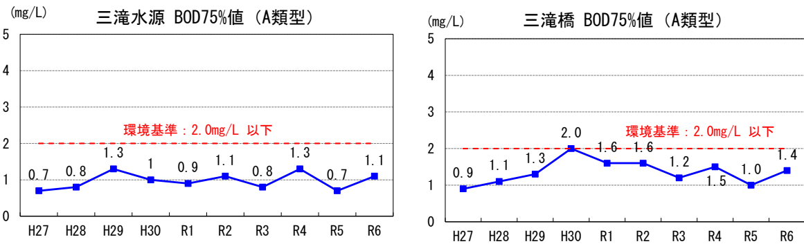
図 2-1 三滝川 みたき BOD75%値経年変化 (赤線は環境基準値を示す)
