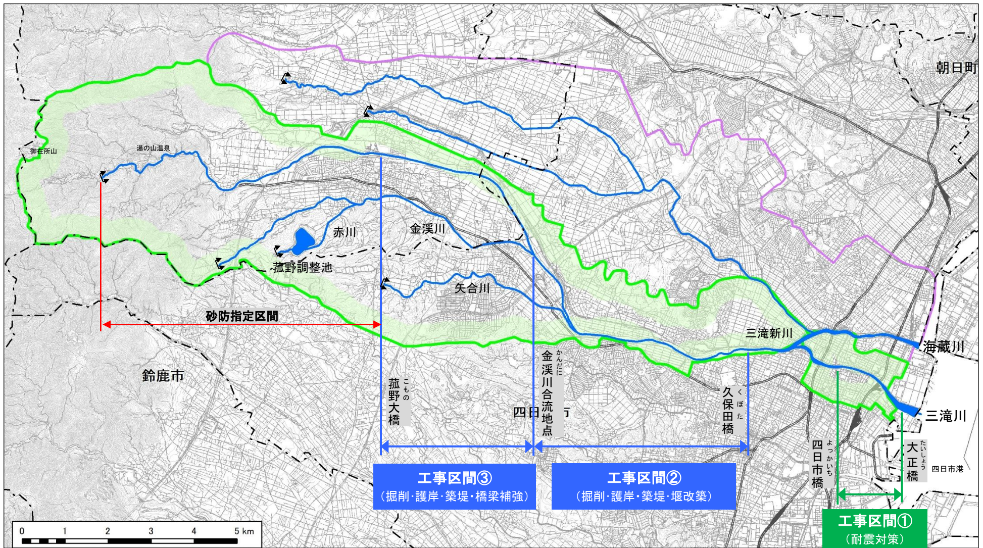
図 河川工事の施行の箇所位置図
